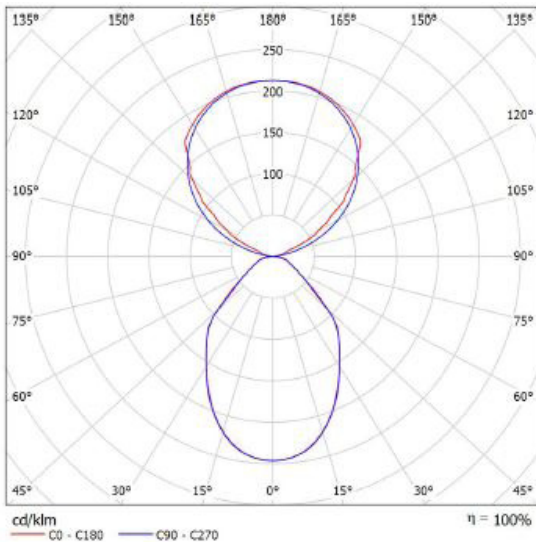
Lichtverteilungskurve H-Fuss 4000K asymmetrisch (LVK)
